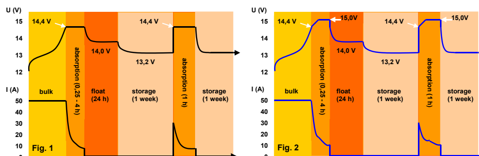
Courbes de charge : jusqu'à tension de gavage (fig.1), et au-delà (fig.2)
